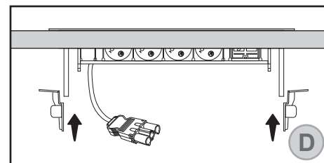
הדק/י את ידיות הנעילה על ידי החדרתם למסילות והידוקן מתחת למשטח כלפי מעלה בחוזקה.
