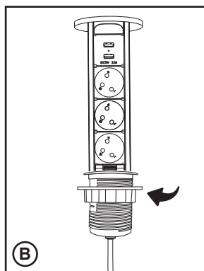
הסר/י מה- Innera Torre את טבעת הנעילה על ידי סיבוב הטבעת עם כיוון השעון.
