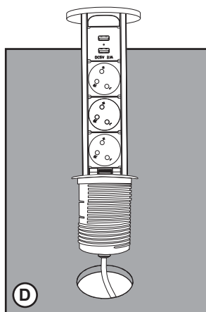
החדר/י את ה- Innera Torre לתוך החור.
