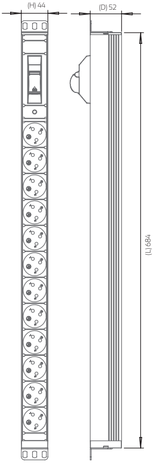
שרטוט להמחשה: דגם EPI2ILM
